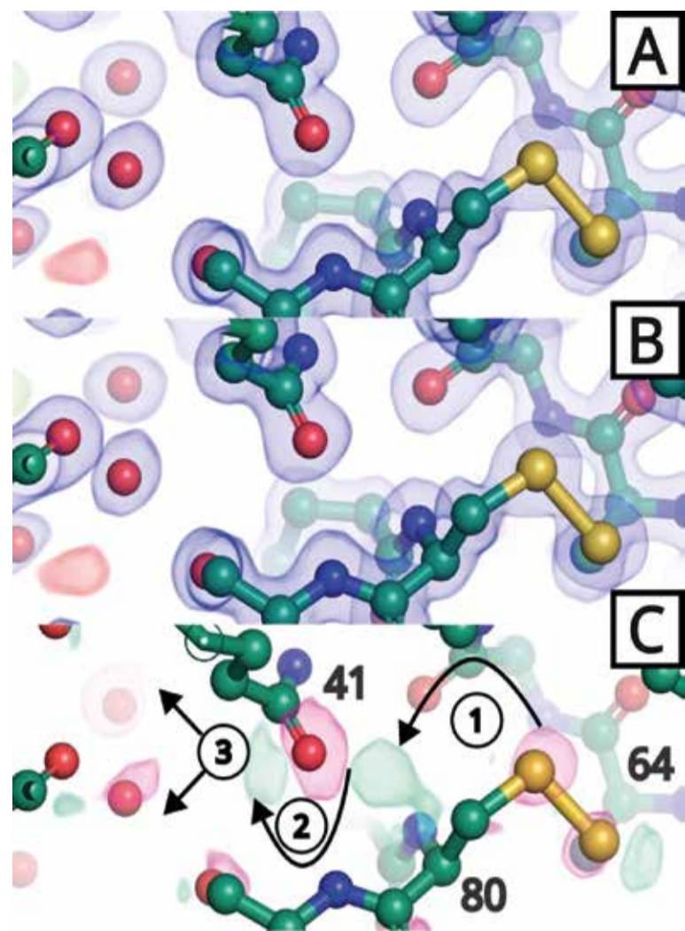
FIGURA 3. RUPTURA de un puente disulfuro— Código de colores: rojo para el oxígeno, verde para el carbono, amarillo para el azufre y azul para el nitrógeno (los hidrógenos no suelen verse en estos modelos). En [A], se muestran los resultados de una primera colecta de datos, el modelo atómico y su densidad electrónica ( nubes en color azul). En [B], igual que en [A], pero este es el producto de una segunda colecta de datos sobre el mismo cristal, con mayor exposición a los rayos X. En [C], se ilustra cómo se ve el daño por radiación, restando la densidad electrónica entre colectas. Ahora las nubes en cian y magenta son similares a las nubes verdes y rojas de la figura anterior. La distinción es que indican cambios ocurridos entre las colectas. Los átomos de azufre del puente disulfuro, formado por los residuos 64-80, tienen menor densidad electrónica en la segunda colecta de datos, lo que sugiere su ruptura. El residuo 80 adopta una nueva posición (1), provocando un reajuste en el residuo 41 (2), y desplazando dos moléculas de agua cercanas (3).
